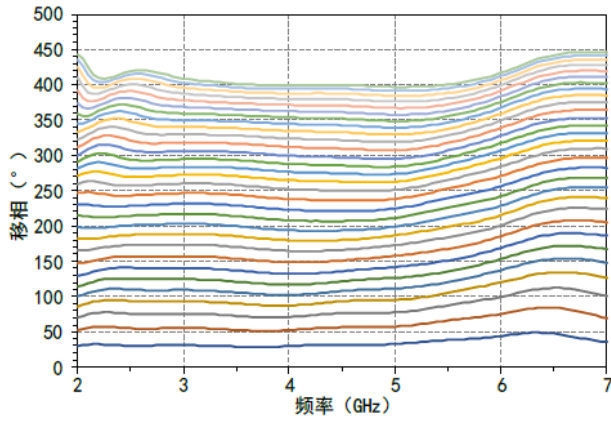
移相VS频率 (Vt=0.5V~15V)
