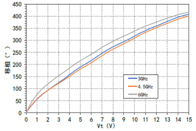
移相 VS Vt
