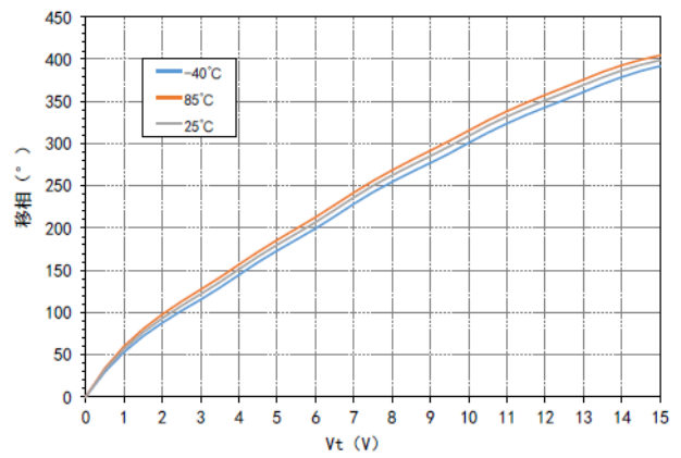
移相 VS Vt@4.5GHz
