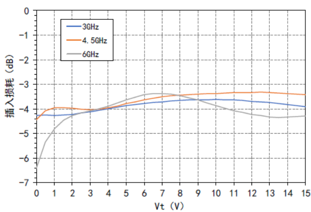
插入损耗VS Vt
